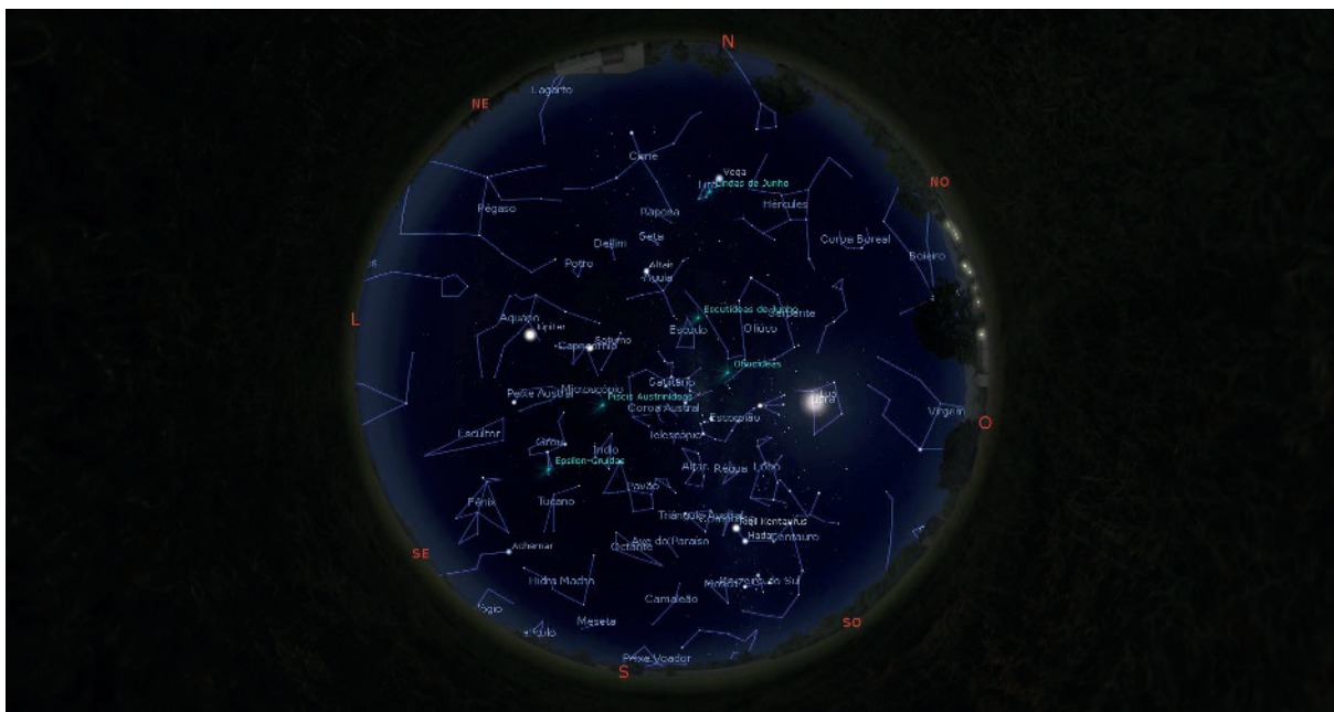
Imagem do céu em Campinas, São Paulo, à 1 hora.
