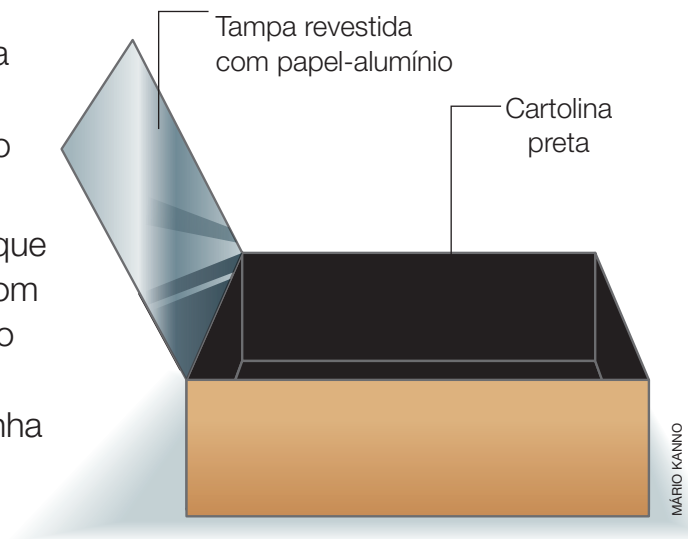
Representação esquemática da montagem do forno solar. (Imagem sem escala; cores fantasia.)
