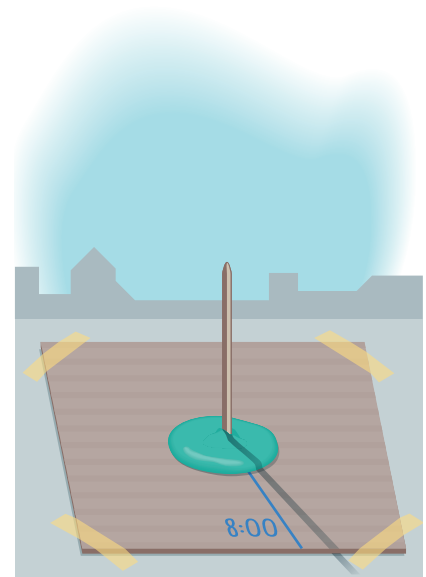
Representação esquemática de um gnômon. (Imagem sem escala; cores fantasia.)
