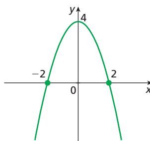
Gráfico 4. Cada elemento do domínio (no eixo x ) tem uma única imagem correspondente no contradomínio (no eixo y ).
