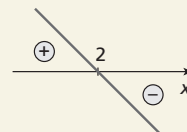
Sinal de g
