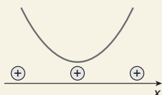
Sinal de g
