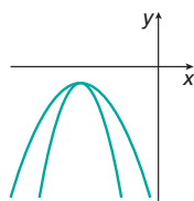
Parábolas com vértice no 3º quadrante e que não interceptam o eixo x .
