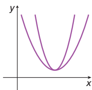
Parábolas com vértice no 1º quadrante e que não interceptam o eixo x .
