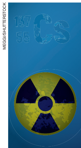
Isótopo radioativo cézio-137.
