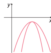
Parábolas com vértice no 4º quadrante e que não interceptam o eixo x .
