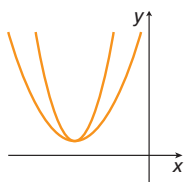
Parábolas com vértice no 2º quadrante e que não interceptam o eixo x .
