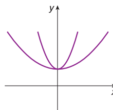
Parábolas com vértice no eixo y e que não interceptam o eixo x .
