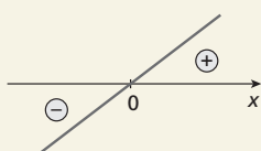
Quadro de sinais
