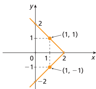
Gráfico 1. Existem elementos do domínio (no eixo x ) que têm mais de um correspondente no contradomínio (no eixo y ).
