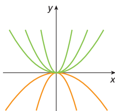
Parábolas com vértice (0, 0) .
