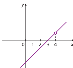
Gráfico 2. Há um elemento do domínio ( x = 4 ) que não tem correspondente no contradomínio (no eixo y ).
