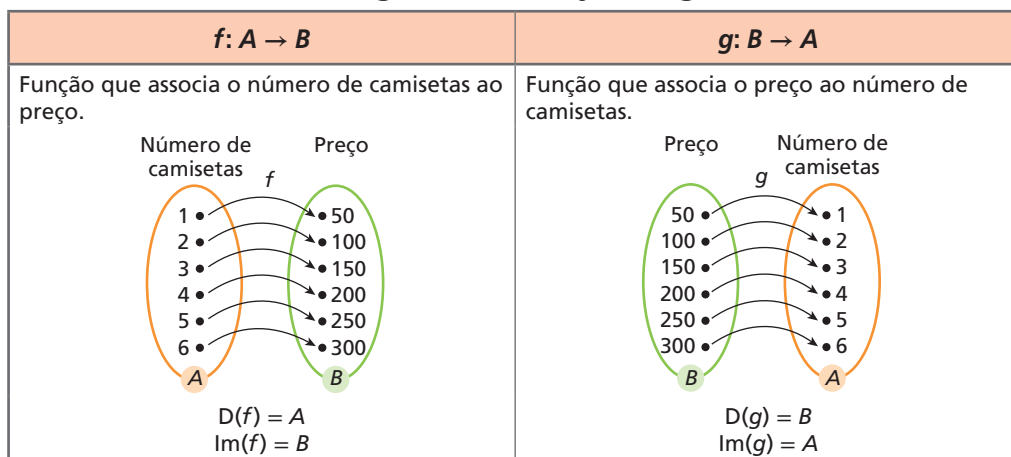
Diagramas das funções f e g
