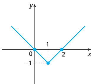
Gráfico 3. Cada elemento do domínio (no eixo x ) tem uma única imagem correspondente no contradomínio (no eixo y ).
